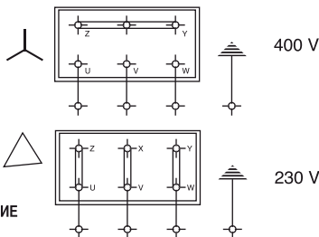
Fig. 1 (Fig. 1) ثلاثي الخطوط الرسم البياني / 1 / Рис. 1 Дارة المثلث : 230 / فولت Дارة النجمة : 400 / فولت
